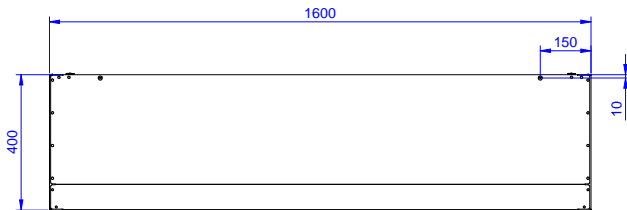
Boven aanzicht
