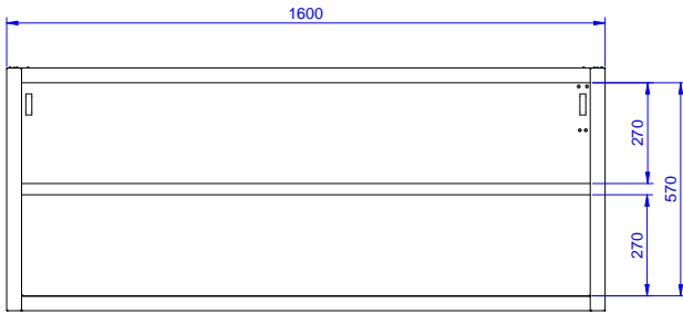
Front aanzicht
